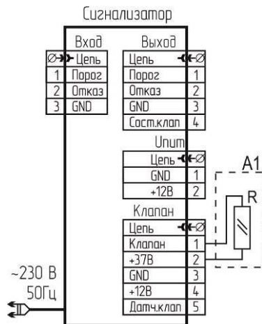
Рисунок В.3 – Схема включения сигнализатора СЗ-2-2В без клапана
