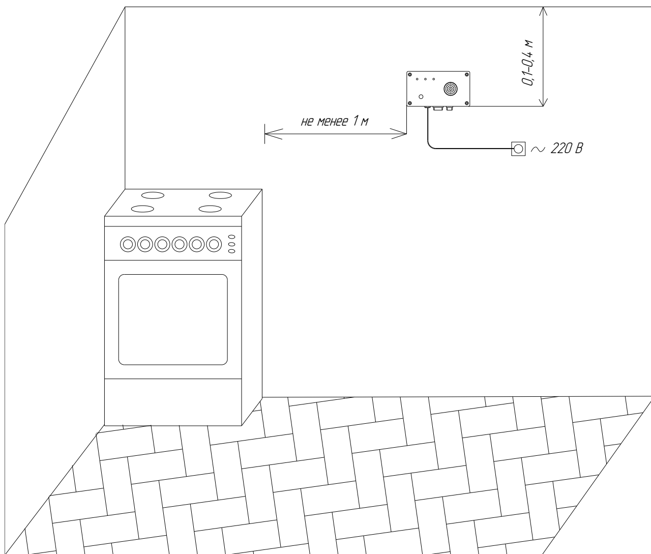
Рисунок 3 - Рекомендуемое местоположение ГС АВУС-М
