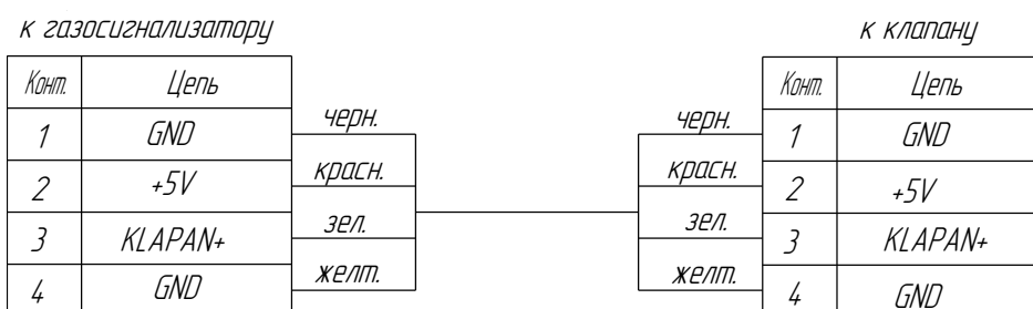
Рисунок Б.2 – Для модификации ПИЖМ.425431.003, ПИЖМ.425431.005.
